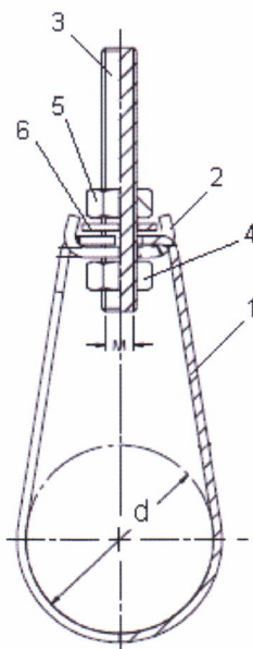
Rys. 2 Konstrukcja uchwyty typu ZP
