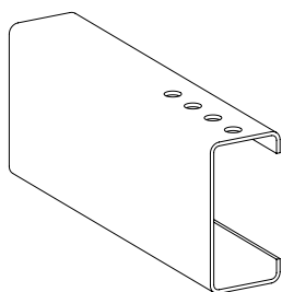
Rys. 2-1 Słup S3H/VS3H
