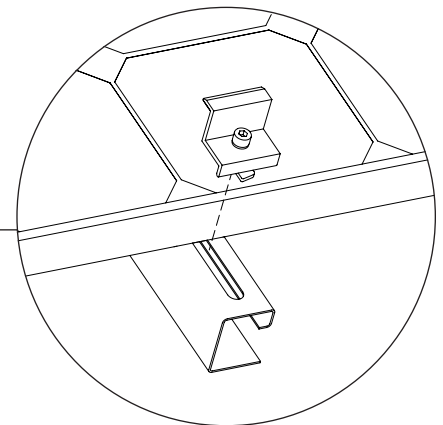
Rys. 4-6 Przykręcenie klemy końcowej VA/VC
