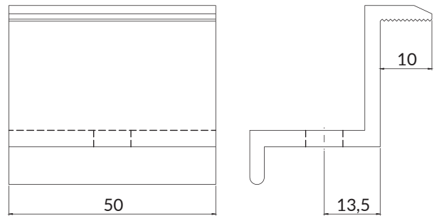
Rys. 4-1 Klema końcowa VA/VC
