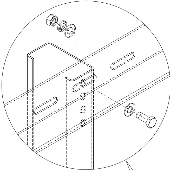
Rys. 3-3 Skręcenie profilu nośnego ze słupem z wykorzystaniem zestawu śrubowego G.1 VNZ
