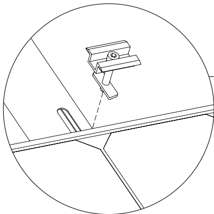
Rys. 4-4 Przykręcenie klemy wewnętrznej VWA/VWC
