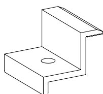
Rys. 2-9 Klema końcowa VA/VC
