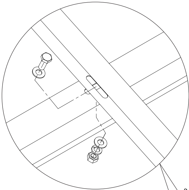
Rys. 3-5 Skręcenie profilu modułowego M15H/VM15H z profilami nośnymi N3H/VN3H z wykorzystaniem zestawu śrubowego G.1 VNZ
